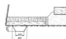
Схема водотливной канавки
