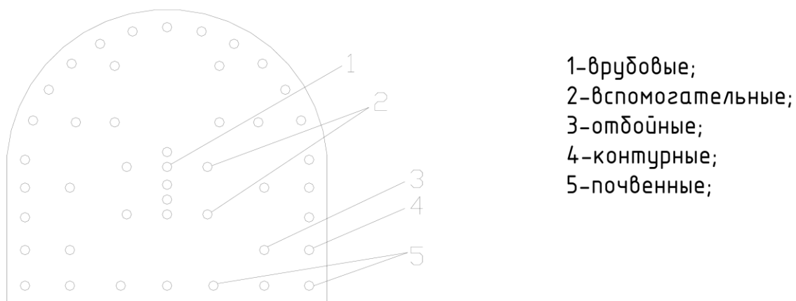
Рис. 2. Схема размещения шпуров
